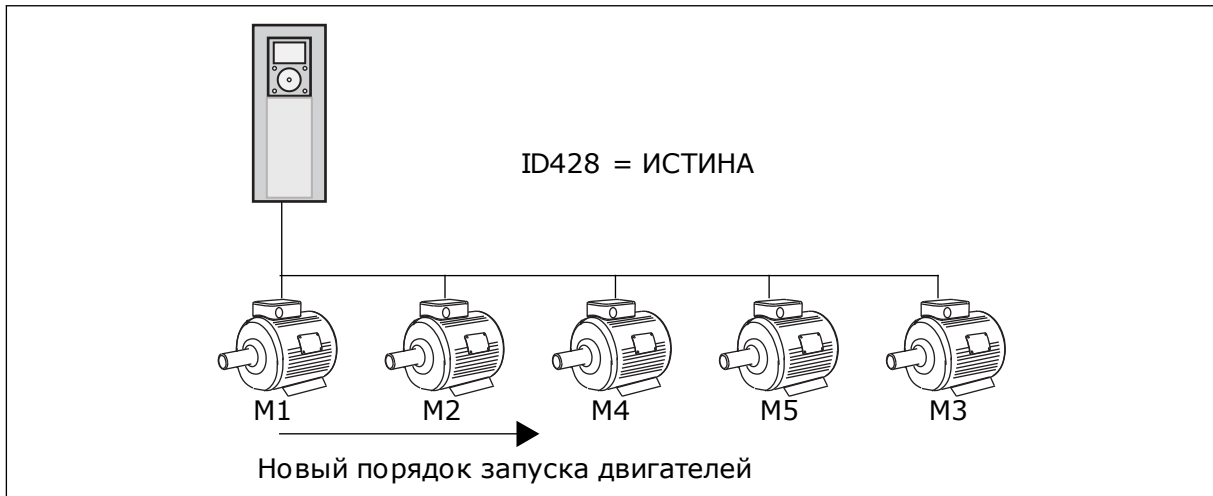
Рис. 47: Логика блокировки 3
