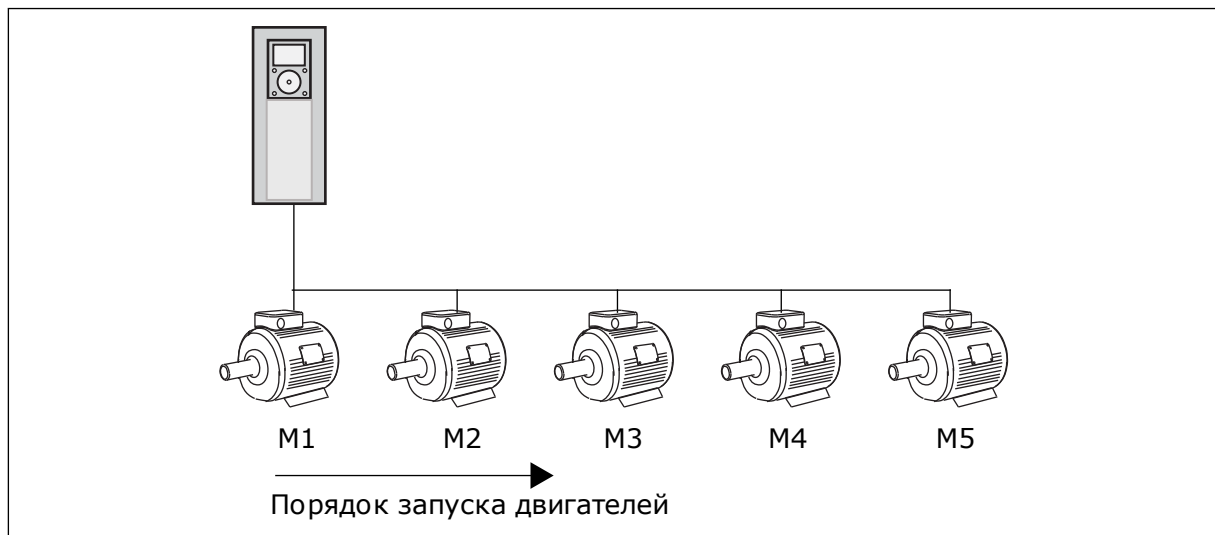
Рис. 45: Логика блокировки 1
