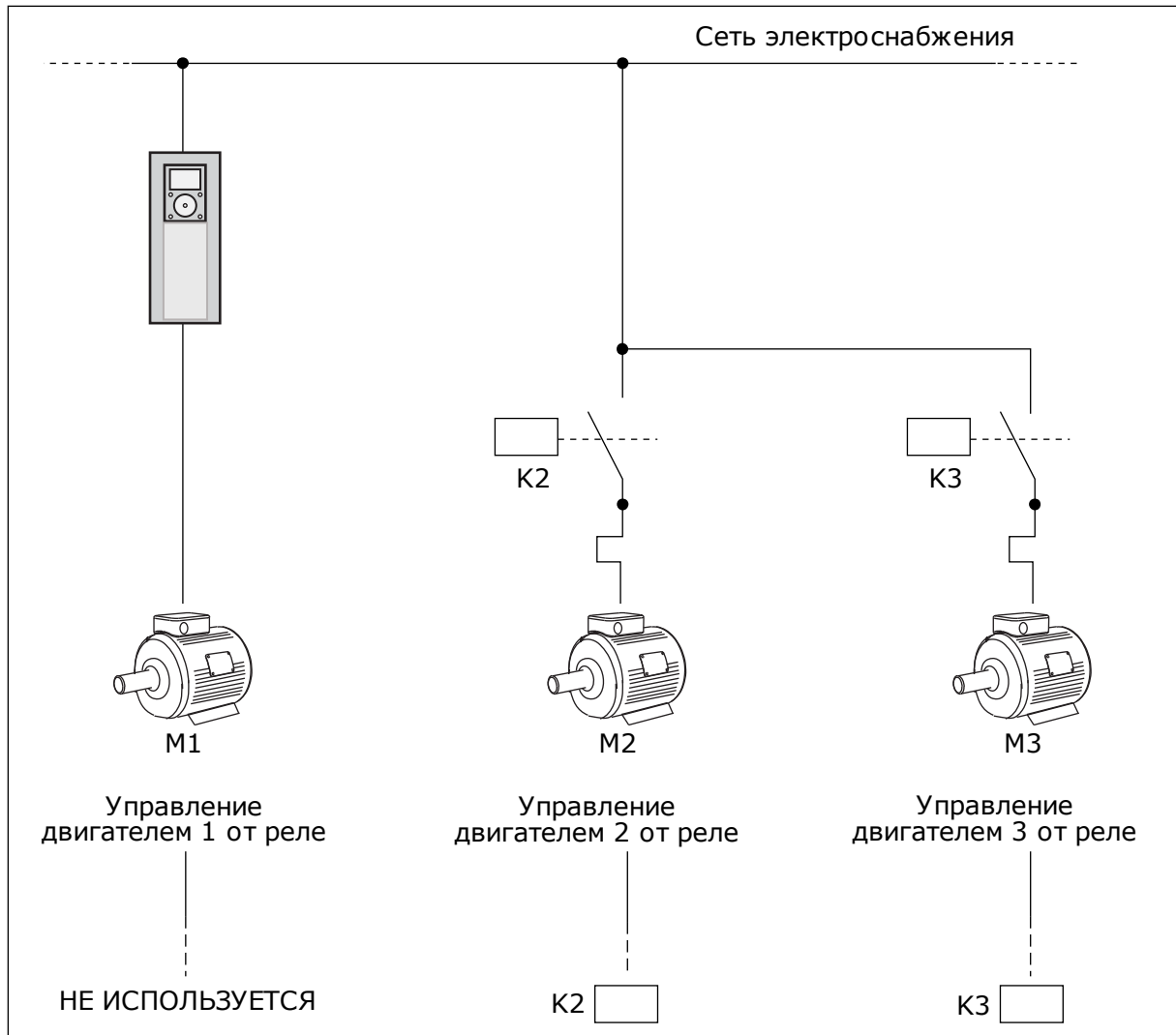
Рис. 48: Выбор 0
