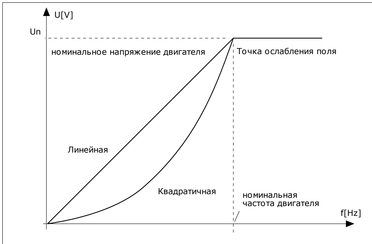
Рис. 13: Линейное и квадратичное изменение напряжения двигателя
