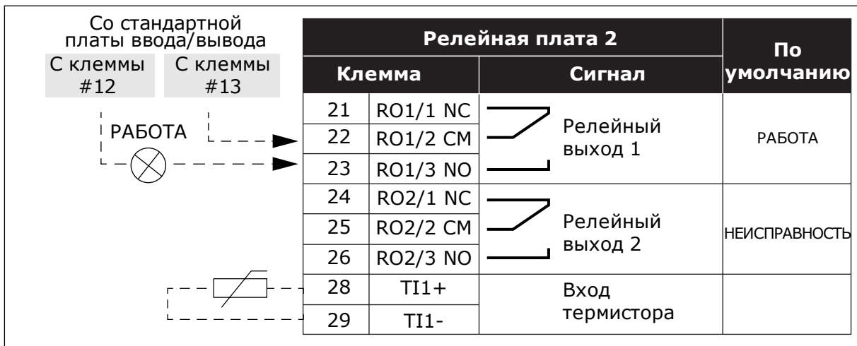
Рис. 6: Пример цепей управления релейной платы 2
