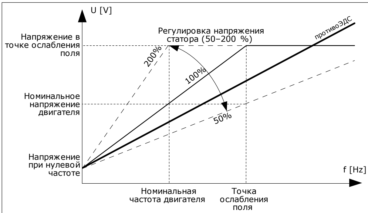
Рис. 14: Регулировка напряжения статора
