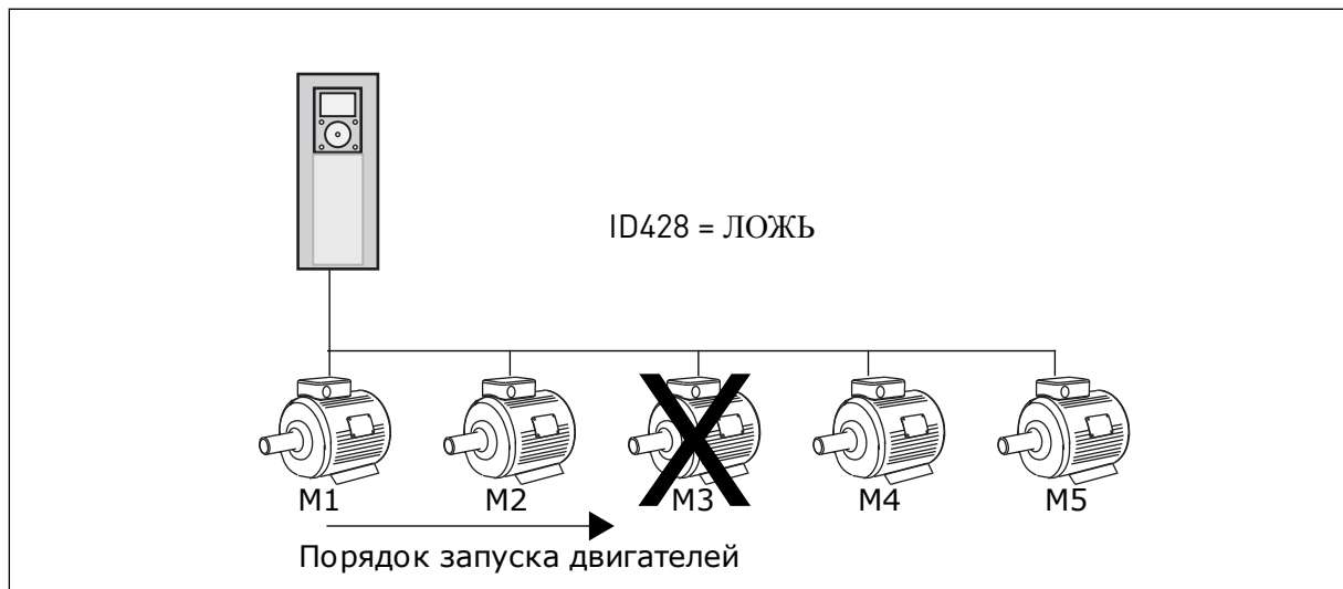
Рис. 46: Логика блокировки 2
