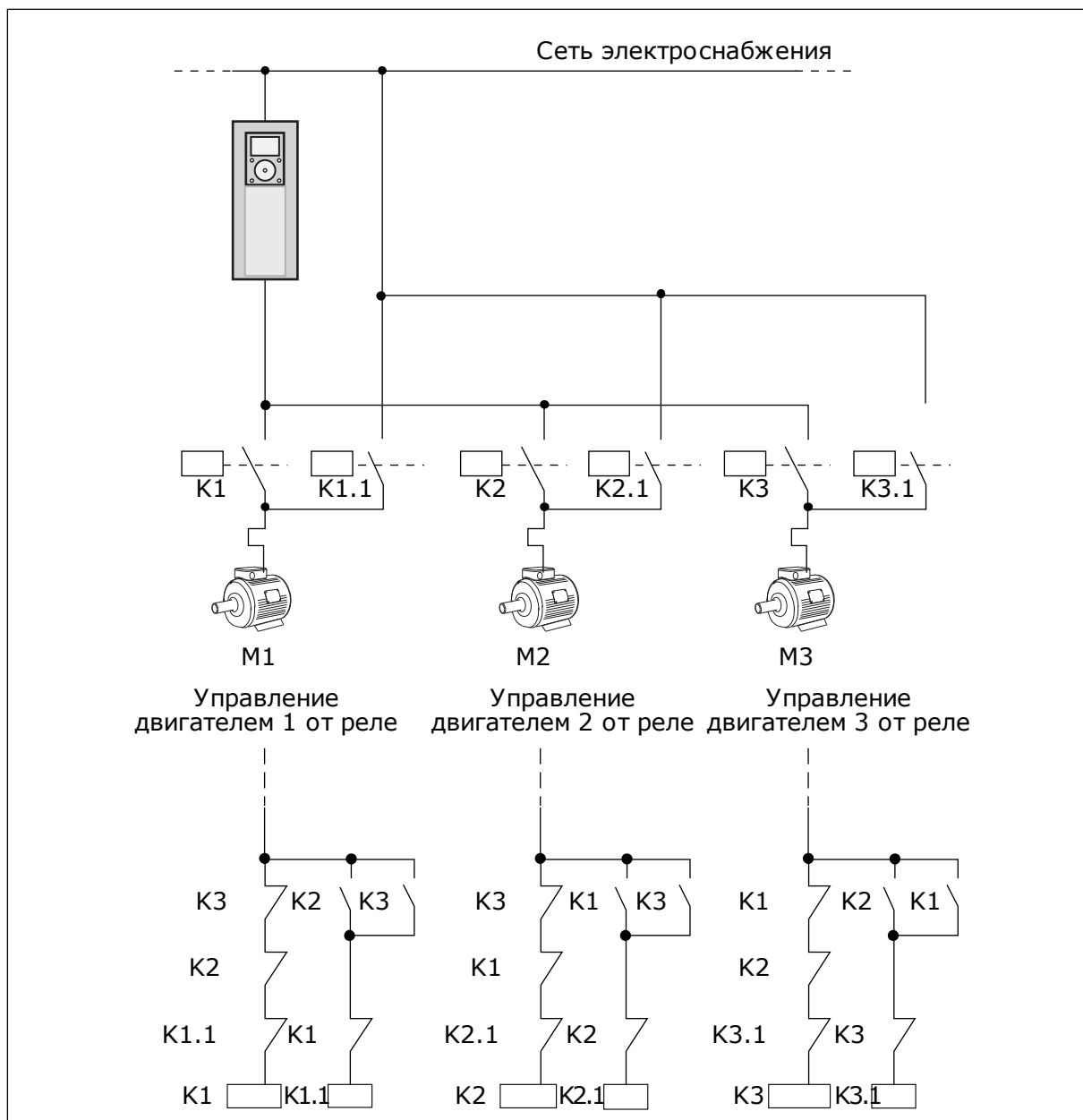
Рис. 49: Выбор 1
