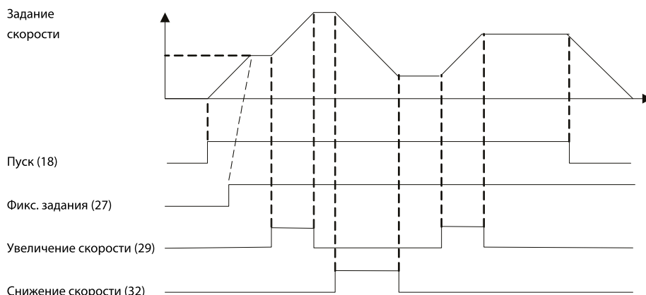
Рисунок 41: Увеличение/снижение скорости
