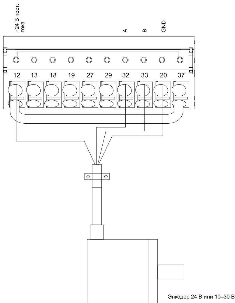
Рисунок 46: Конфигурация проводки для энкодера
