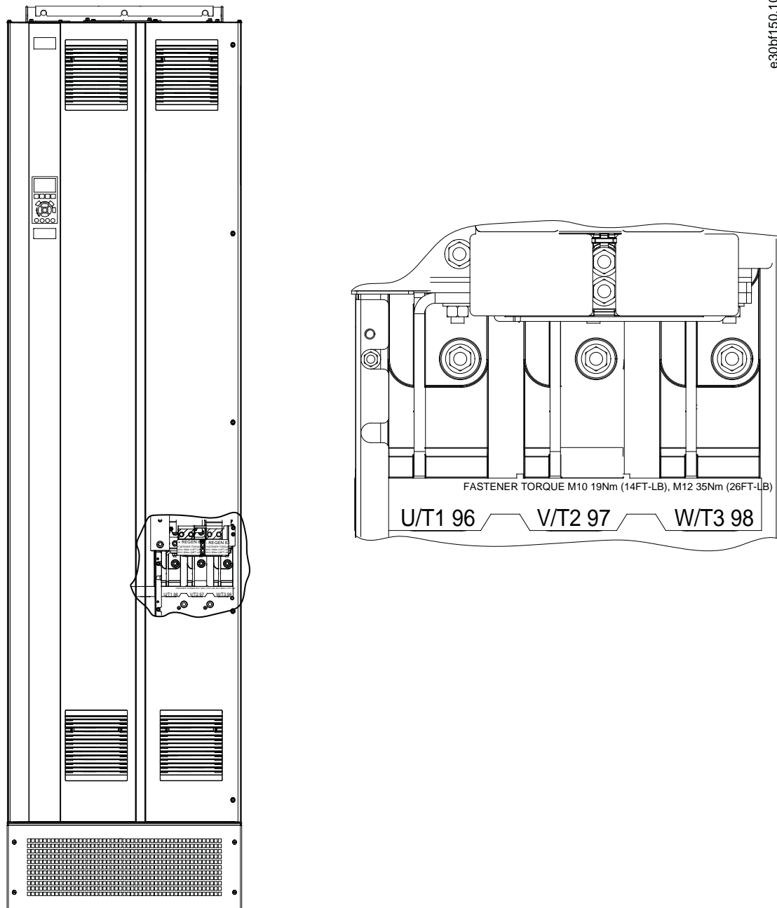
Рисунок 19: Клеммы подключения двигателя пер. тока (показан корпус E1h).
