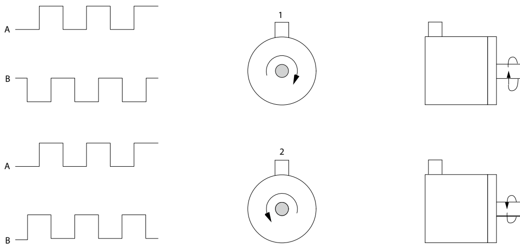
Рисунок 45: Определение направления вращения энкодера
