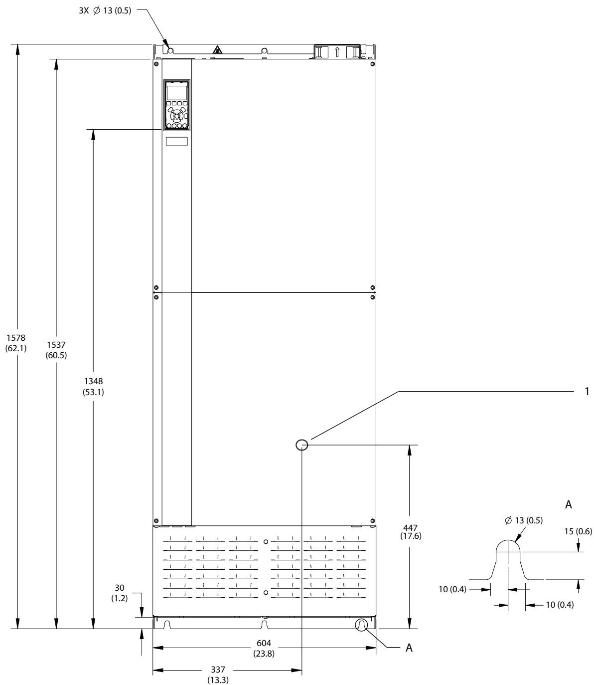
Рисунок 65: Вид спереди E4h
