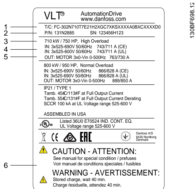
Рисунок 8: Паспортная табличка изделия (для корпуса E2h, пример)
