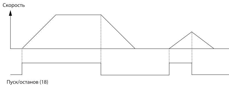
Рисунок 42: Команда пуска/останова с Safe Torque Off
