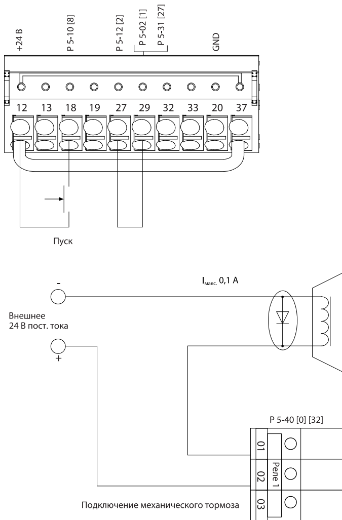
Рисунок 47: Конфигурация проводки для крутящего момента и предела останова
