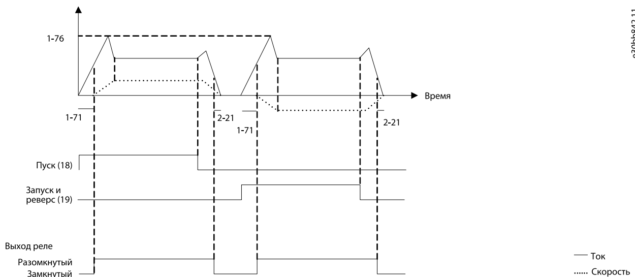
Рисунок 44: Управление механическим тормозом
