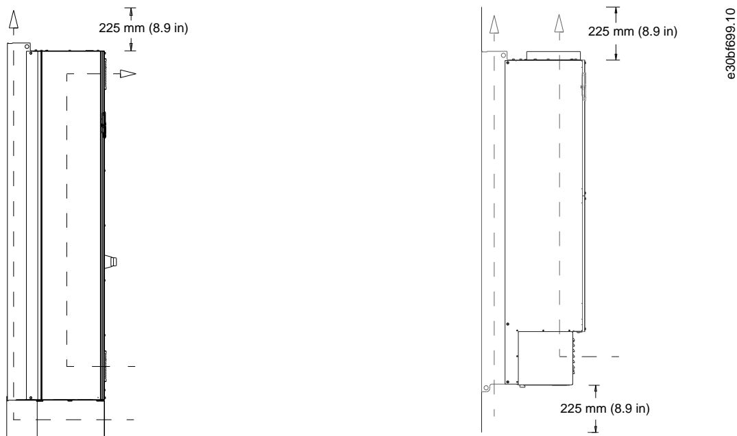
Рисунок 69: Циркуляция воздуха через корпуса E1h/E2h (слева) и E3h/E4h (справа)
