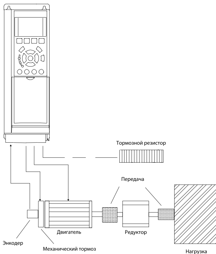
Рисунок 40: Базовая настройка замкнутого контура управления скоростью
