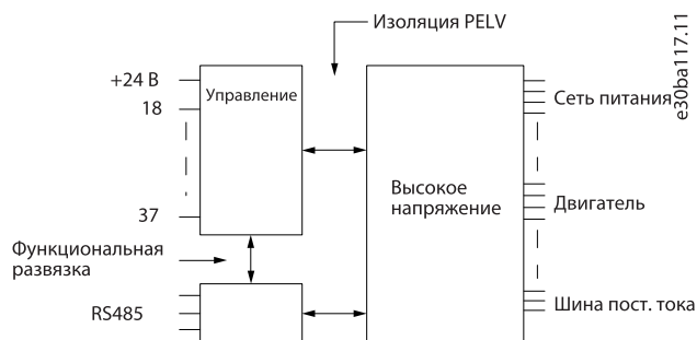
Рисунок 52: Изоляция PELV
