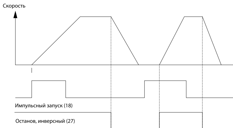
Рисунок 43: Импульсный запуск/останов, инверсный
